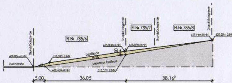
Geländeschnitt M = 1:1000
