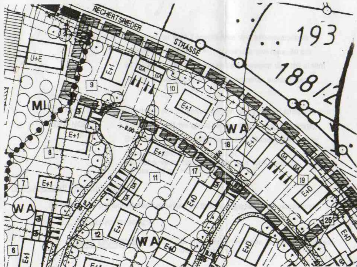
DECKBLATT 2 - FESTSETZUNG M 1:1000
