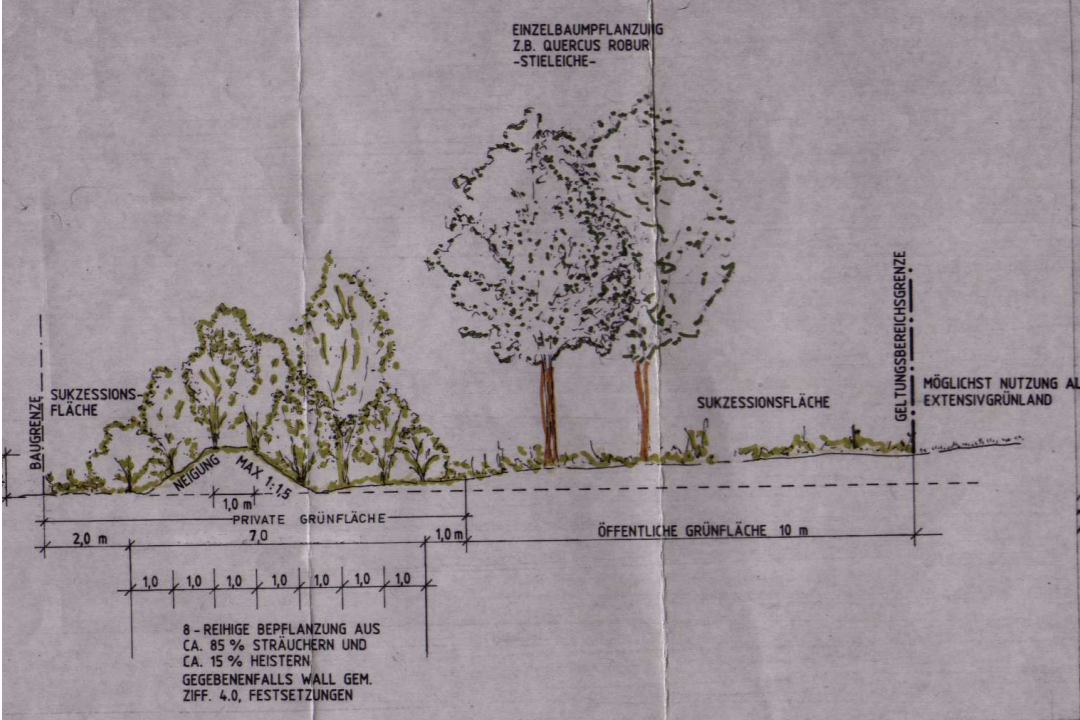
SCHEMASCHNITT A-B M=1:100 WALLSCHÜTTUNG UND RANDBEPLANZUNG ENTLANG DER NORDOSTGRENZE
